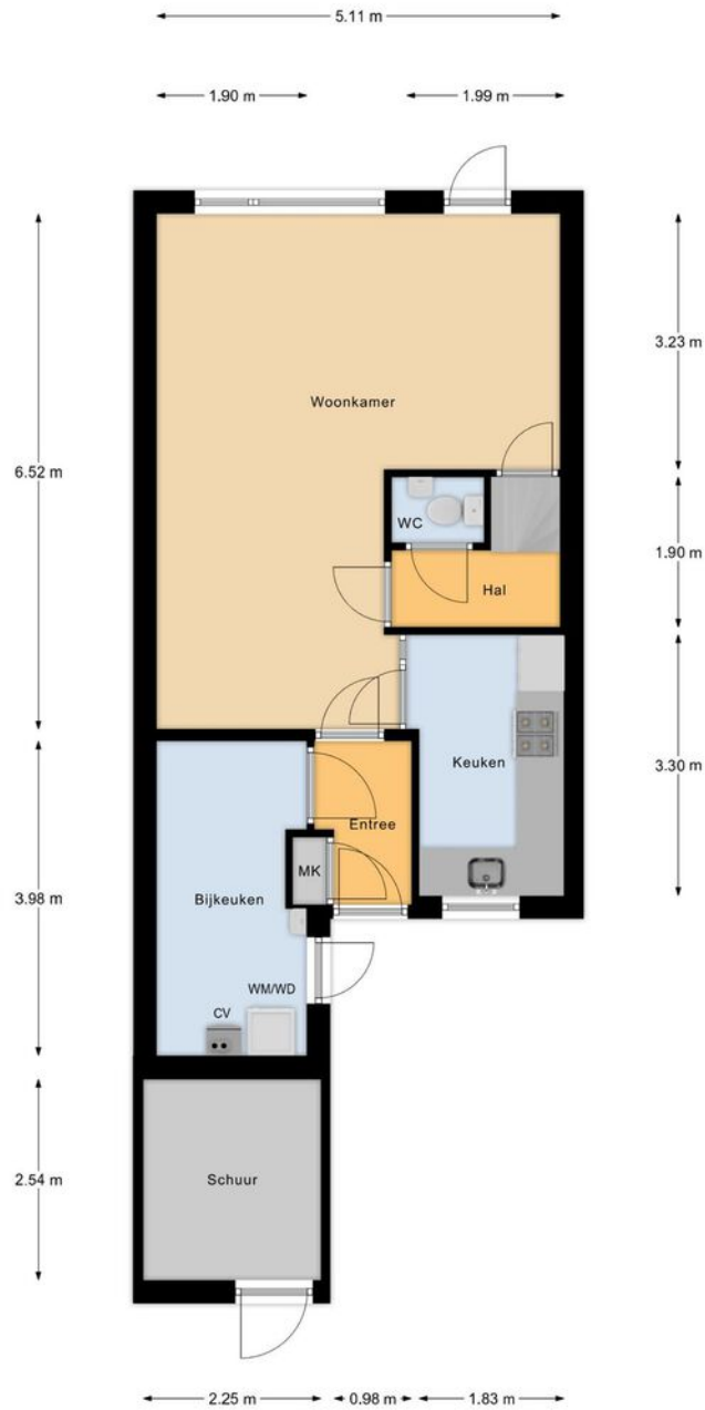
Begane Grond
