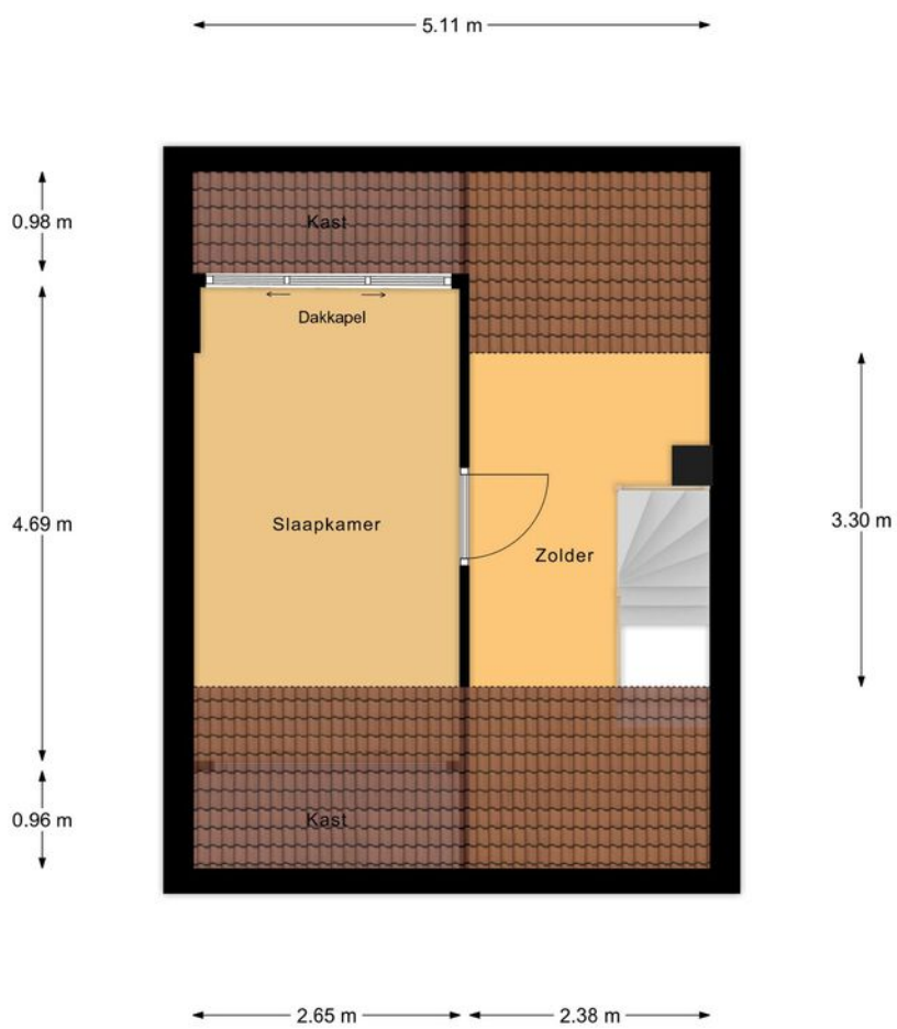
2e Verdieping
