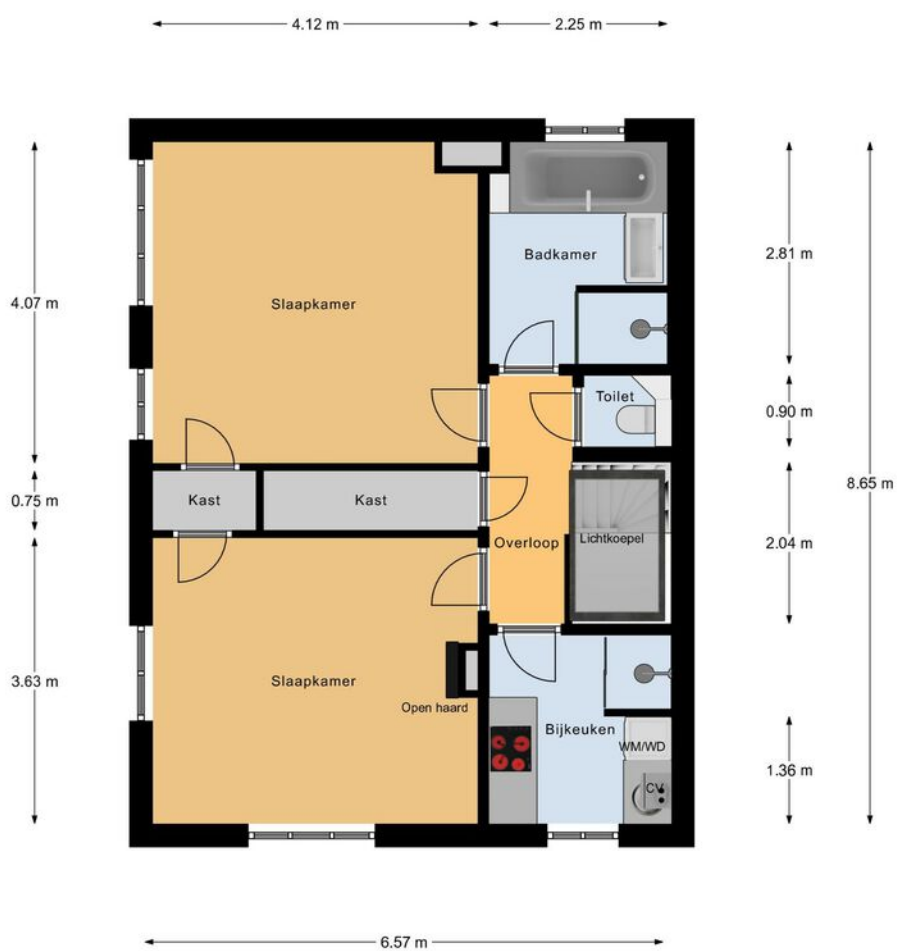
Tweede Verdieping
