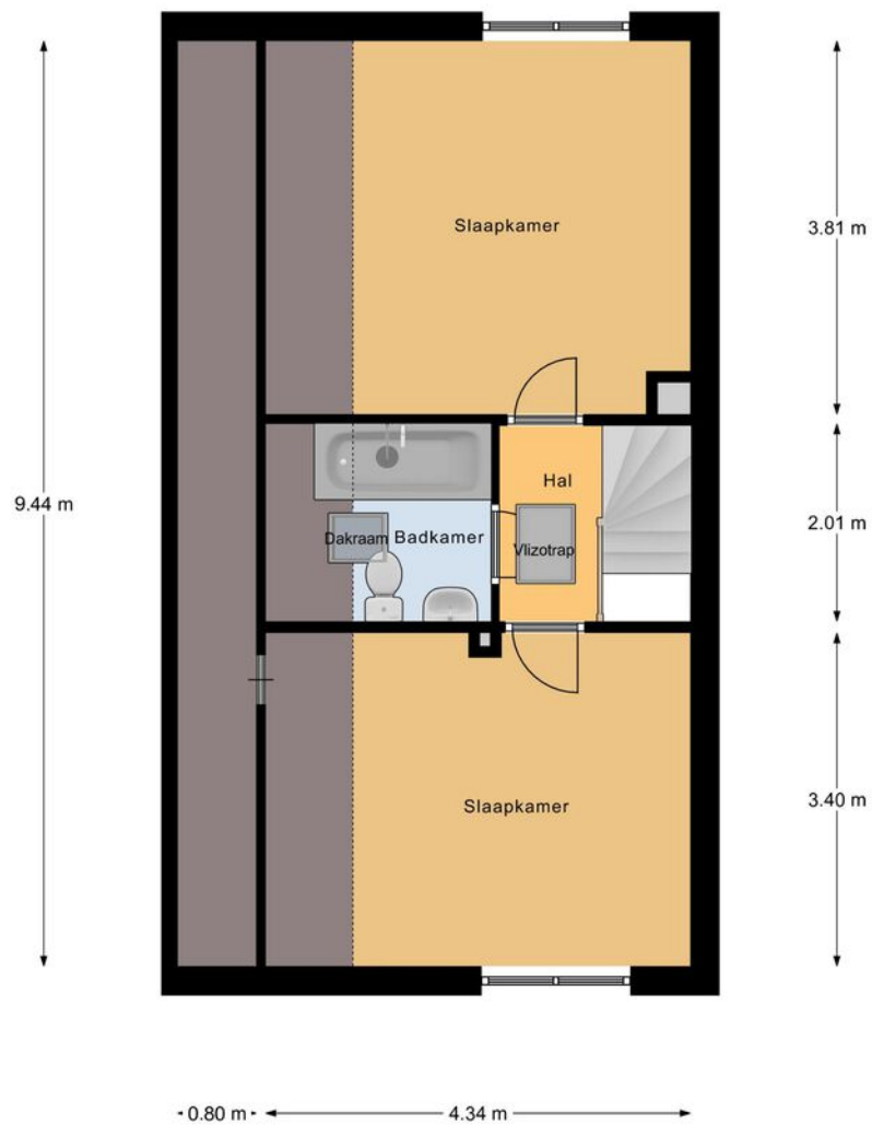
1e Verdieping
